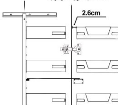
فاصله سبد کوچک از درب
