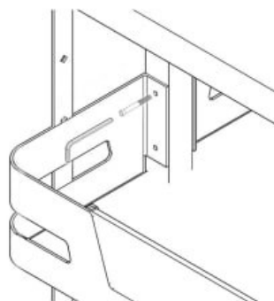
نحوه اتصال سبد به قاب ریل
