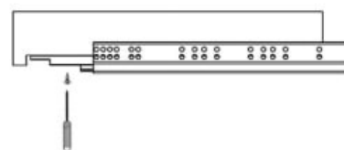
نحوه اتصال ریل به کف
