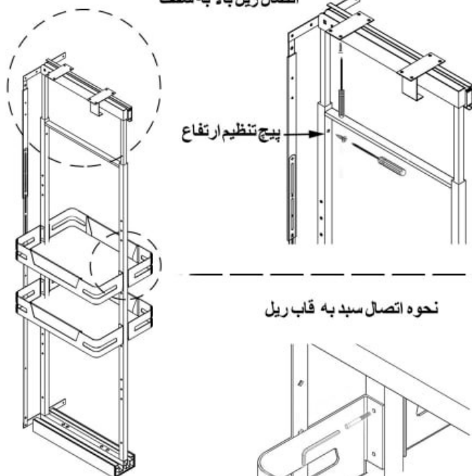
اتصال ریل بالا به سقف
